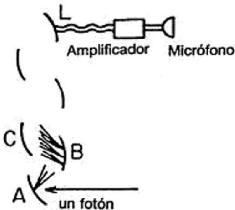
Figura 1. Un fotomultiplicador puede detectar un único fotón. Cuando un fotón incide sobre la placa A, libera un electrón que es atraído por la placa B, cargada positivamente, arrancando más electrones a su vez. Este proceso continúa hasta que miles de millones de electrones inciden sobre la última placa, L, y producen una corriente eléctrica, que es aumentada por un amplificador. Si se conecta un altavoz al amplificador, se oyen clicks de volumen uniforme cada vez que un fotón de un color determinado incide sobre la placa A.
