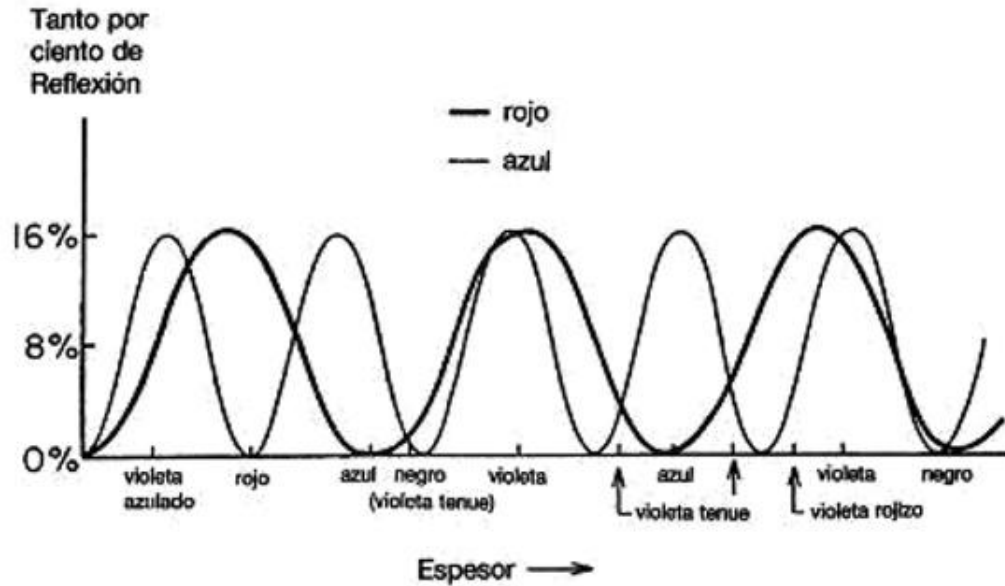
Figura 18. Al aumentar el espesor de la lámina, las dos superficies producen una reflexión parcial de la luz monocromática cuya probabilidad fluctúa cíclicamente desde el 0% al 16%. Puesto que la velocidad de la manecilla imaginaria del cronógrafo es distinta para los distintos colores de luz, el ciclo se repite a velocidades diferentes. Así cuando dos colores puros como rojo y azul inciden sobre la lámina, un espesor determinado reflejará sólo rojo, sólo azul, azul y rojo en proporciones diferentes (lo que produce varios matices de violeta), o ningún color (negro). Si la lámina es de espesor variable, como una gota de aceite extendiéndose en un charco fangoso, todas las combinaciones tendrán lugar. Con la luz del Sol, que contiene todos los colores, tendrá lugar todo tipo de combinaciones, lo que produce montones de tonalidades.
