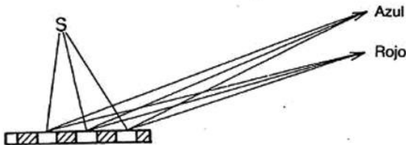
Figura 27. Una red de difracción con surcos a la distancia adecuada para la luz roja, también funciona para otros colores si el detector se coloca en un lugar diferente.
