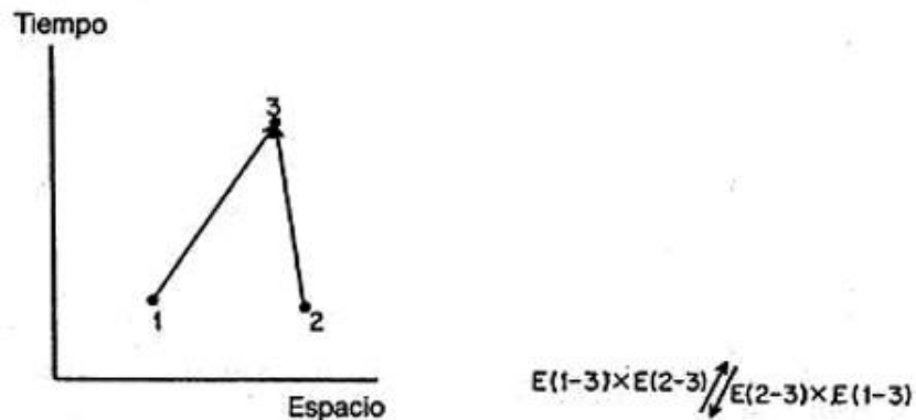
Figura 72. Si dos electrones (con la misma polarización) intentan ir al mismo punto del espacio-tiempo, la interferencia es siempre negativa debido a los efectos de polarización: las dos flechas idénticas — E(1 \text{ a } 3) \times E(2 \text{ a } 3) y E(2 \text{ a } 3) \times E(1 \text{ a } 3) — se restan para dar una flecha final de longitud nula. La aversión de dos electrones a ocupar el mismo lugar del espacio-tiempo se denomina «Principio de Exclusión» y es el responsable de la gran variedad de átomos en el universo.
