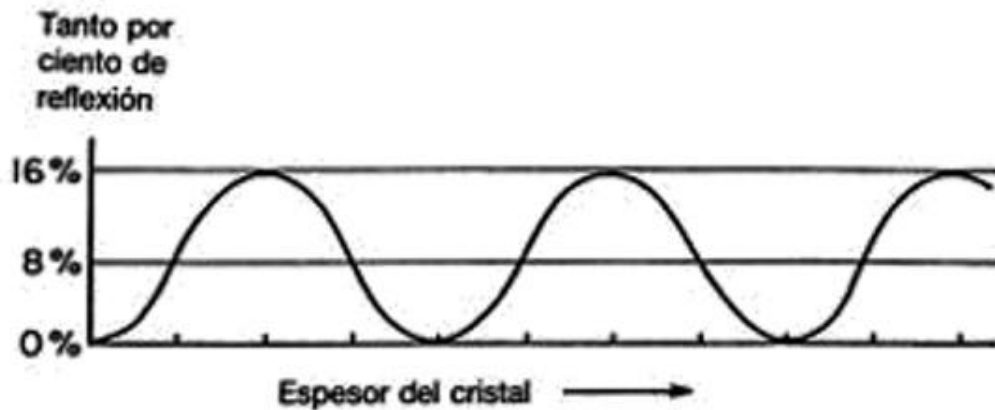
Figura 5. Los resultados de un experimento que mide cuidadosamente la relación entre el espesor de una lámina de cristal y la reflexión parcial, demuestran la existencia de un fenómeno llamado «interferencia». Al aumentar el espesor del cristal, la reflexión parcial experimenta un ciclo de repetición desde 0 al 16%, sin síntomas de extinción.
