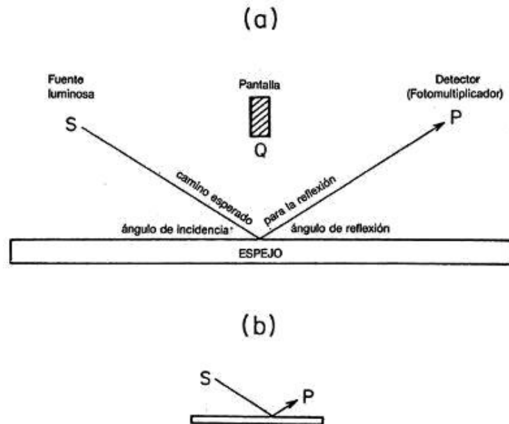
Figura 19. El punto de vista clásico del mundo dice que un espejo reflejará la luz allí donde el ángulo de incidencia iguale al de reflexión, incluso si la fuente y el detector están en niveles diferentes, como en (b).
