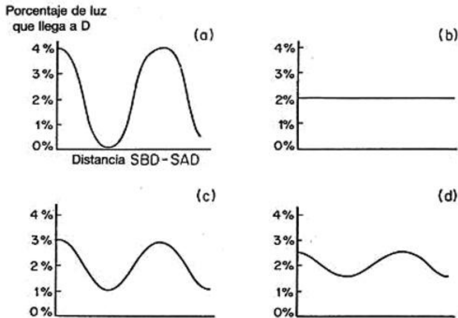
Figura 51. Cuando no existen detectores en A o B, existe interferencia —la cantidad de luz varía de cero al 4% (a) —. Cuando hay detectores en A y B que son fiables al 100%, no existe interferencia —la cantidad de luz que alcanza D es una constante, el 2% (b) —. Cuando los detectores en A y B no son fiables al 100% (es decir, cuando a veces no hay nada colocado en A o B que pueda detectarse), existen tres posibles condiciones finales —A y D se disparan, B y D se disparan, y D se dispara solo—. La curva final es una mezcla, formada de contribuciones de cada una de las posibilidades finales. Cuando los detectores en A y B son menos fiables, hay mayor interferencia presente. Así los detectores en el caso (c) son menos fiables que en el caso (d). El principio referente a la interferencia es: La probabilidad de cada una de las distintas condiciones finales posibles debe de ser calculada de manera independiente sumando flechas y elevando al cuadrado la longitud de la flecha final; luego, las diversas probabilidades se suman de la manera normal.
