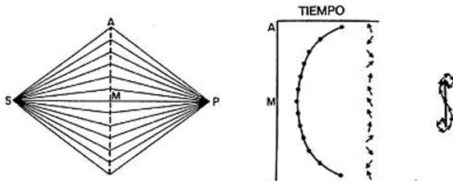
Figura 35. El análisis de todos los caminos posibles de S a P se ha simplificado y se incluyen sólo los de doble línea recta (en un único plano). El efecto es el mismo que para el más complicado caso real: existe una curva de tiempos con un mínimo, de donde procede la contribución mayor a la flecha final.
