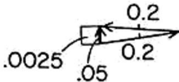
Figura 12. La flecha final, cuyo cuadrado representa la probabilidad de reflexión por una lámina de cristal extremadamente delgada, se dibuja sumando la flecha de reflexión frontal con la flecha de reflexión posterior. El resultado es casi nulo.
