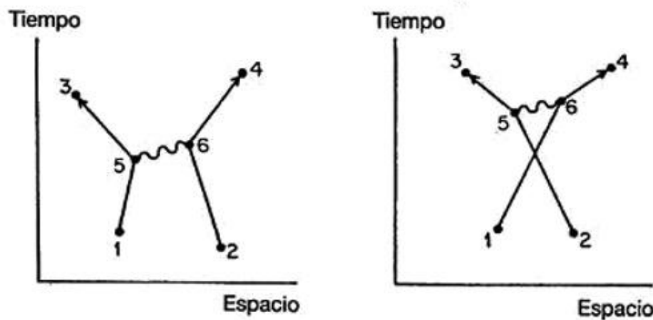
Figura 60. Dos caminos «caminos alternativos» por los que el suceso de la Fig. 59 puede tener lugar: en cada caso se emite un fotón en 5 y se absorbe en 6. Las condiciones finales de ambas alternativas son las mismas que en los otros casos —dos electrones entran y dos electrones salen— y estos resultados son indistinguibles de los de otras alternativas. En consecuencia, las flechas para estos «caminos alternativos» se deben sumar a las flechas de la Fig. 59 para obtener una mejor aproximación a la flecha final del suceso.
