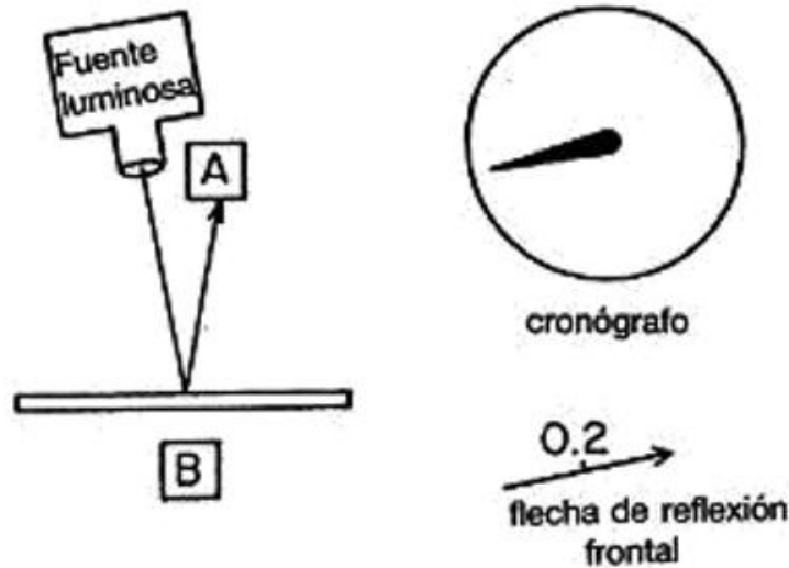
Figura 10. En un experimento que mide la reflexión por dos superficies, podemos decir que un único fotón puede llegar a A por dos caminos —por vía de la superficie frontal o de la posterior—. Para cada camino se dibuja una flecha de longitud 0,2, con su dirección determinada por la manecilla de un «cronógrafo» que cronometra al fotón cuando se mueve. La flecha de «reflexión frontal» se dibuja en el sentido opuesto al que señala la manecilla del cronógrafo cuando se detiene.
