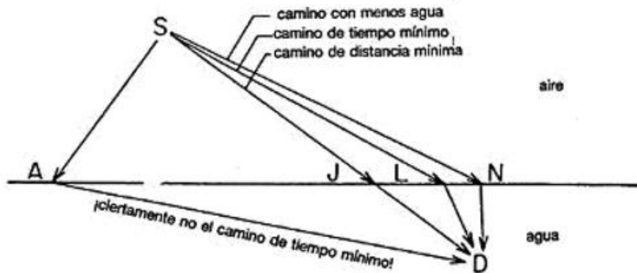
Figura 30. Encontrar el camino de tiempo mínimo la luz es análogo a encontrar el camino de tiempo mínimo para un socorrista que corriendo y luego nadando rescata a una víctima que se está ahogando: el camino más corto tiene demasiada parte con agua; el camino de menor porción de agua tiene demasiada parte con tierra; el camino de menor tiempo es un compromiso entre los dos.
