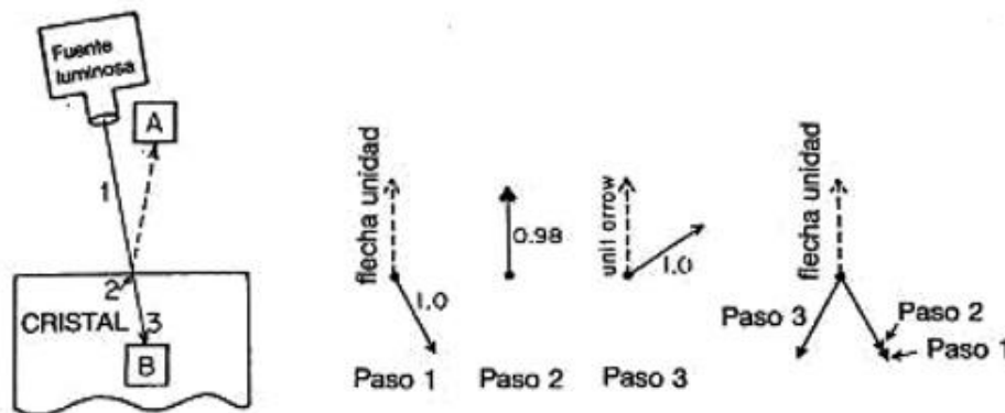
Figura 41. La transmisión a través de una superficie también se puede dividir en tres pasos, con una reducción y/o giro en cada uno. Una flecha de longitud 0,98 tiene un cuadrado de aproximadamente 0,96, representando una probabilidad de transmisión del 96% (lo que combinado con la probabilidad de reflexión del 4%, da cuenta del 100% de luz).
