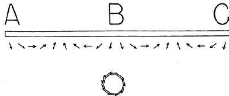
Figura 25. Para comprobar la idea de que realmente existe reflexión en los extremos del espejo (pero que se cancela) hacemos un experimento con un trozo grande de espejo colocado en si ti o equivocado para la reflexión de S a P. Este trozo de espejo se di vi de en secciones mucho más pequeñas, de manera que el tiempo entre un camino y el siguiente no sea muy diferente. Cuando se suman todas las flechas, no conducen a ninguna parte: forman un círculo y su suma es muy próxima a nada.
